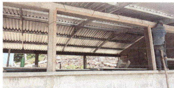
Foto 2: Ventana; en proceso de detallado
